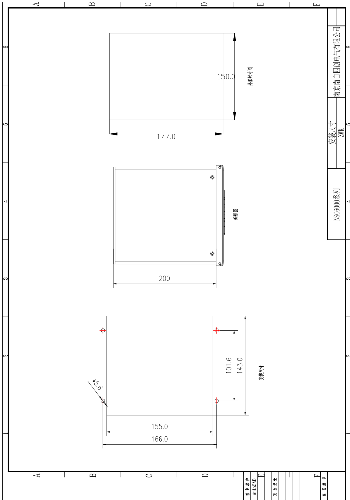
图 4: NSC 620U 数字式系列数字式电动机保护装置安装尺寸图:
