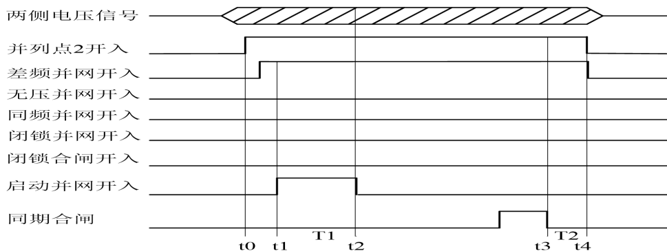
图 4-3 开入操作时序图
