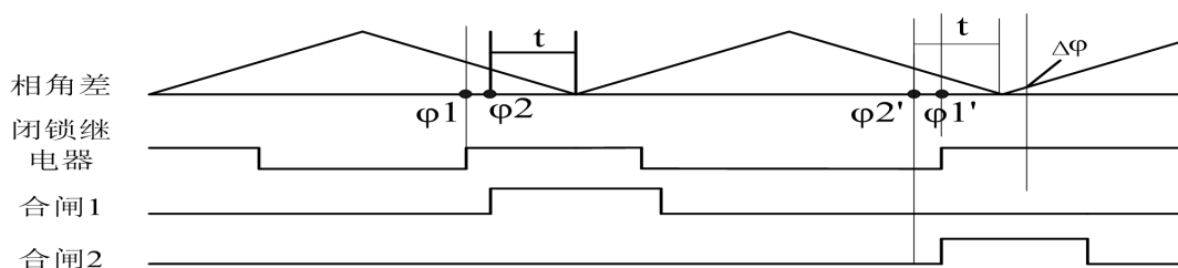
图 4-8 合闸回路中存在同步闭锁继电器
