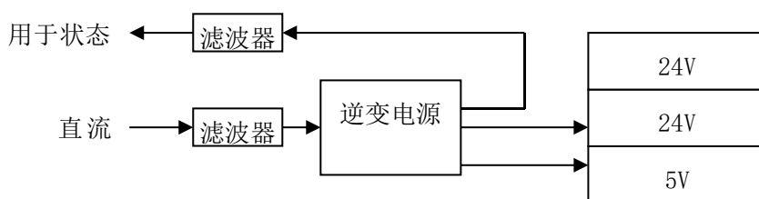
图 3-3 电源模块原理示意图
