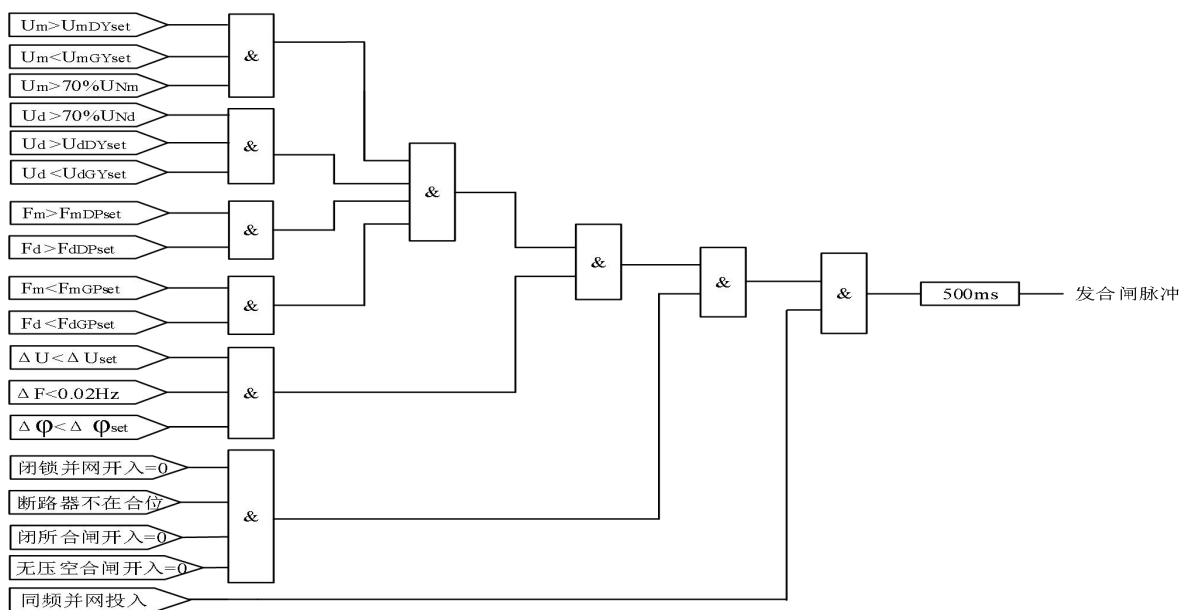
图 4-2-2 同频并网逻辑框图
