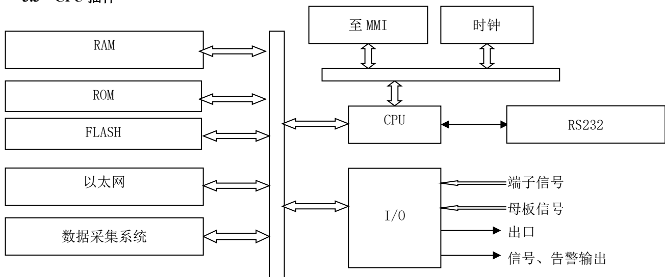
图 3-1 CPU 模块原理示意图
