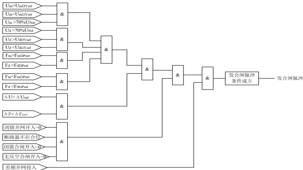
图 4-2-1 差频并网逻辑框图
