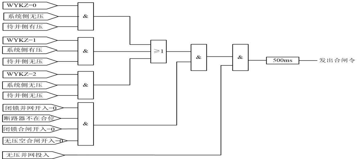
图 4-2-3 无压并网逻辑框图
