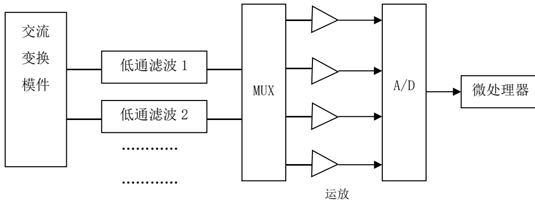
图 3-2 A/D 系统原理示意图
